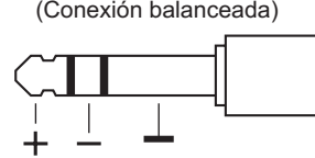
ENTRADA SALIDA/LINK JACK (Conexión balanceada)
