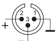
ENTRADA - XLR (Conexión balanceada)
