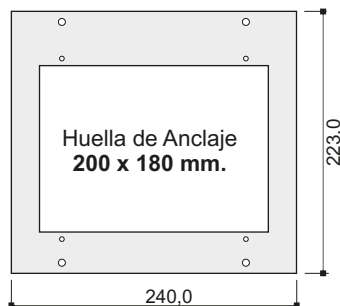
Accesorio opcional IW-500 Montaje empotrado
