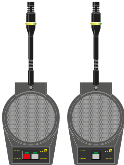
Pupitre Presidente SC-401
