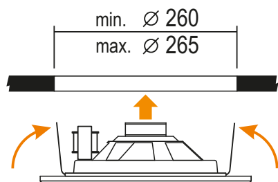
MONTAJE EN FALSO TECHO FALSE CEILING ASSEMBLY
