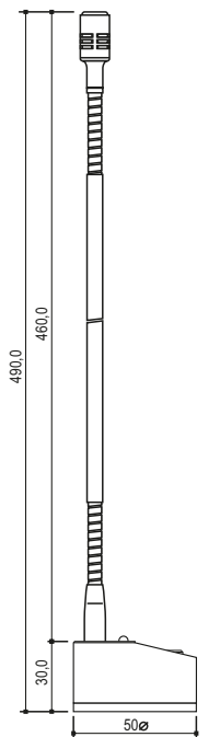
DIMENSIONES EN MILIMETROS
