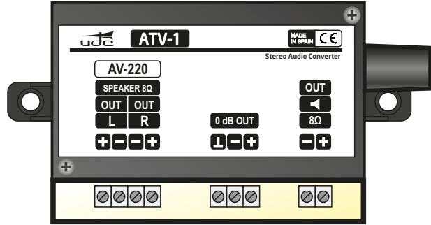
ATV-1 Convertor de línea estereo
