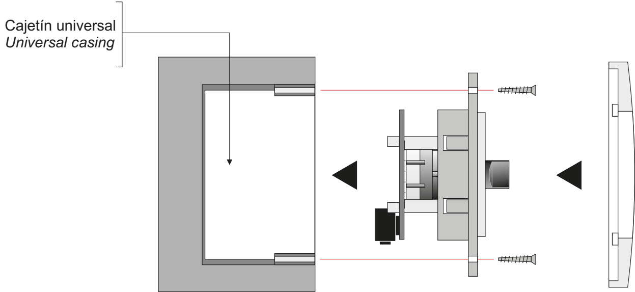
MONTAJE EMPOTRADO FLUSH MOUNTING
